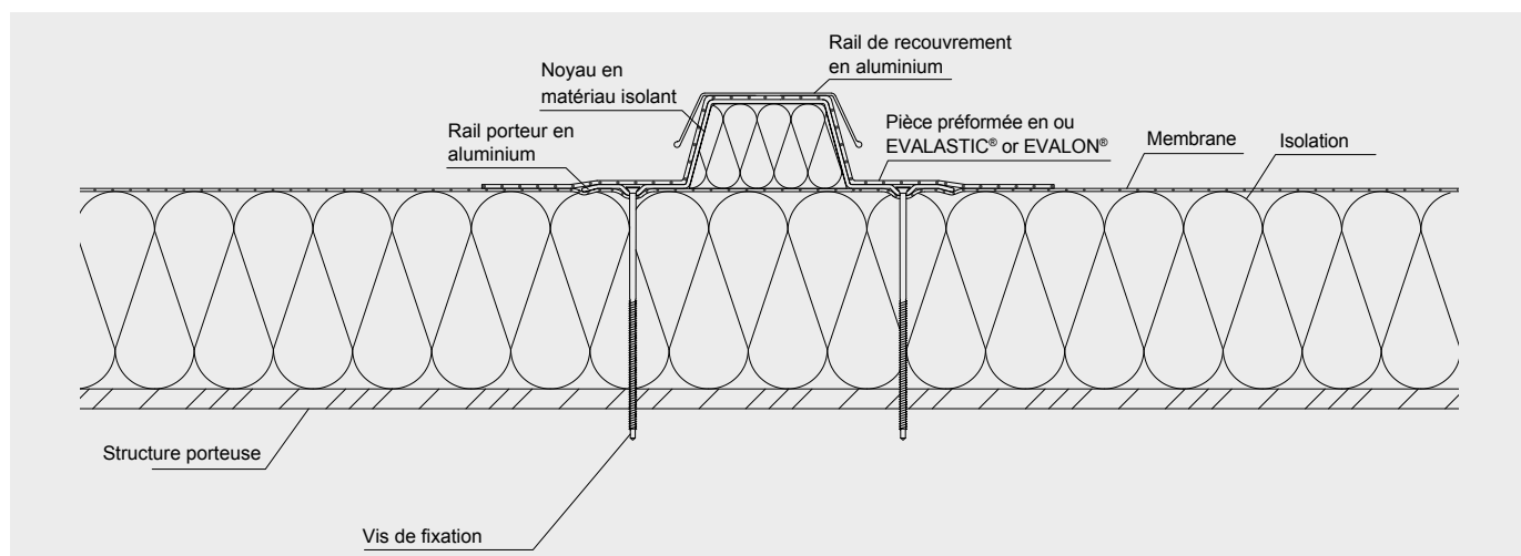
Rail de montage EVATEC® Solar d'alwitra : montage simple sur l'étanchéité de toiture, fixation sûre à l'aide de vis de fixation
