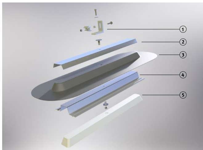
Vue éclatée du rail de montage EVATEC® Solar d'alwitra :
