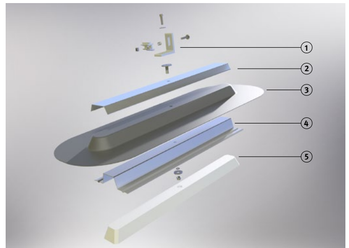
Explosions-Darstellung der alwitra Montageschiene EVATEC® Solar:
