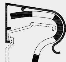
Bitumen-Deckprofil Polymerbitumen-Dachbahn
