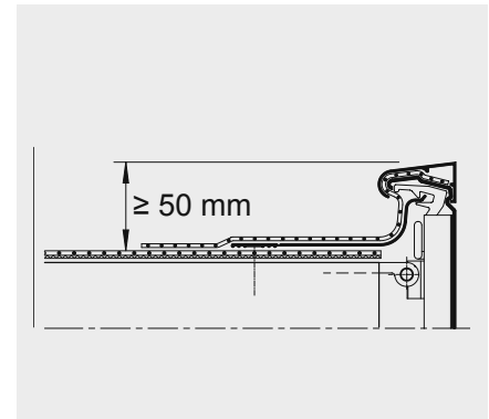
Über 5° Dachneigung
